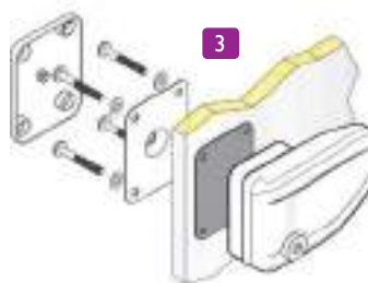
Montage sur la paroi
